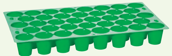
Multitopf-Platte 38 Töpfe 50 x 30 x 6 cm, 38 Töpfe Ø Ø 5,5 cm oben, Ø 3,9 cm unten, ca. 6 mm Bodenloch, PS 0,6 mm Art.-Nr. 10294010, Kt.-Inh. 25
