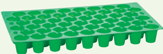
Multitopf-Platte 51 Töpfe 50 x 30 x 5,5 cm, 51 Töpfe Ø Ø 4,6 cm oben, Ø 3,2 cm unten, ca. 6 mm Bodenloch, PS 0,6 mm Art.-Nr. 10294009, Kt.-Inh. 30
